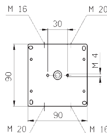
Schalterstirnseite Front view
