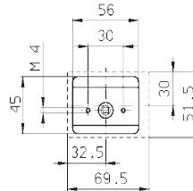
Schalterstirnseite Front view
