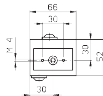
Schalterstirnseite Front view
