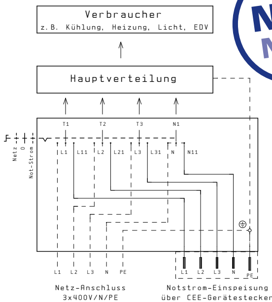
Schaltbild Circuit diagram
